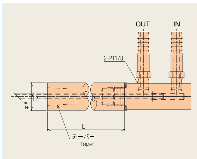
写真はストレートホルダー、分水器、銅パイプのセットです。 Photo shows a set of straight holder, water divider and copper pipe.
